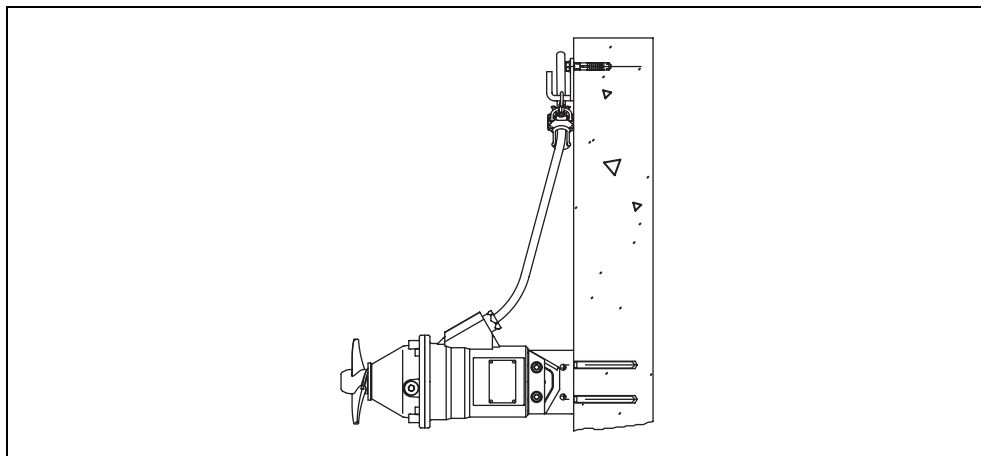
Рис. 5-1: Настенный монтаж
