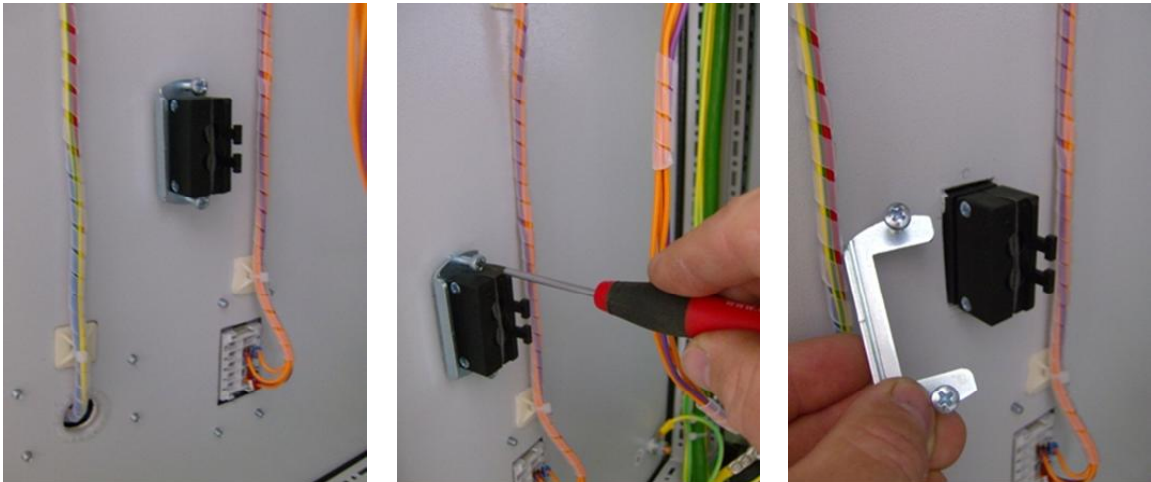
Демонтировать ввод кабеля с боковой стенки
